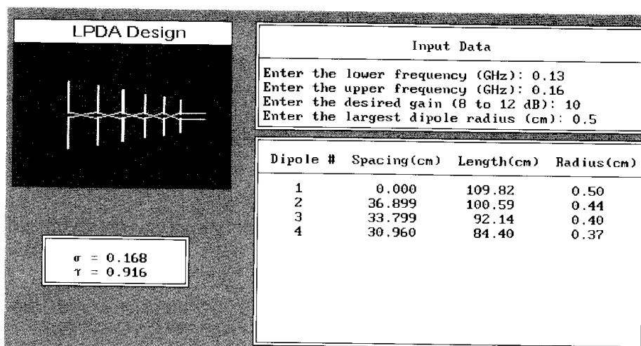
Bild 2: Die untere Tabelle enthält nun alle Maße und Abstände der einzelnen LPDA-Antennenelemente. Der linke, längste Dipol der Anordnung stellt die Nummer 1 dar
