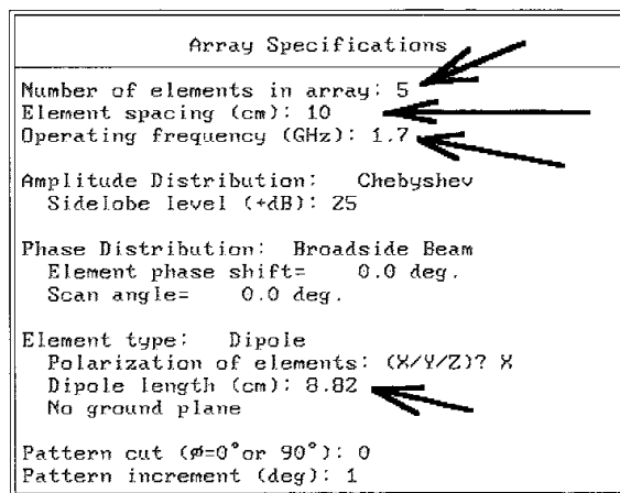
Bild 4: Entwurfsbeispiel für ein lineares Antennenarray. Mit Pfeilen sind die erforderlichen Eingaben markiert. Im Feld „Selected Action“ wählt man die auszugebenden Ergebnisse
